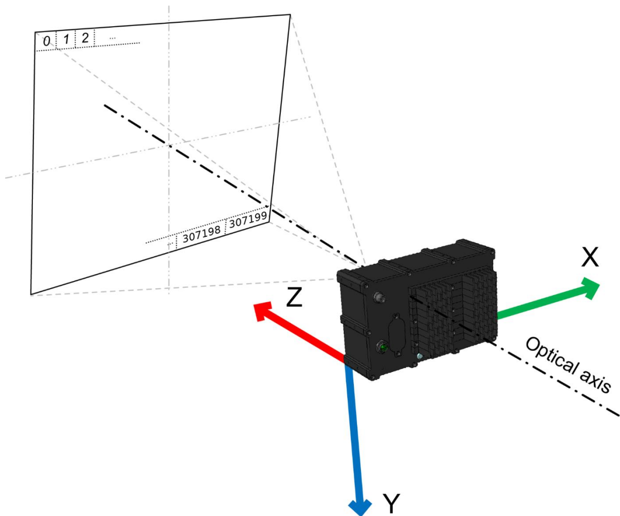
Figure 11-1: TOREO-P650 Default Coordinate System (2)
